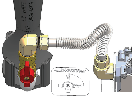
FIGURE 15. Position du gaz naturel, Premier 170 illustré
