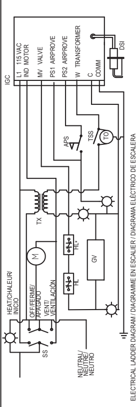
ELECTRICAL CONNECTION DIAGRAM / CONNEXIONS ELECTRIQUES / DIAGRAMA DE CONEXIONES ELECTRICAS
