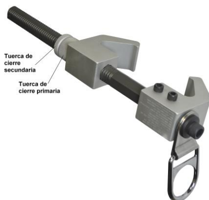
Fig. 3.6 Anclaje de viga vertical (7535)
