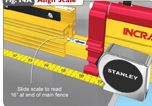
Fig. 14A Align Scale
