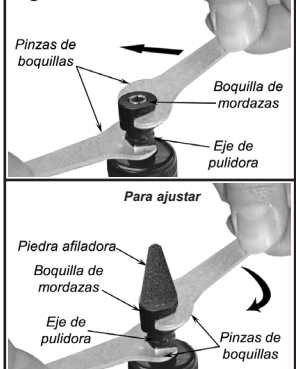
Figura 3 Para aflojar
